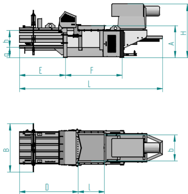
HPK 750 / 950 / 1100 / 1100 K
